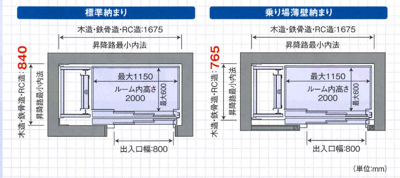
昇降路平面図
